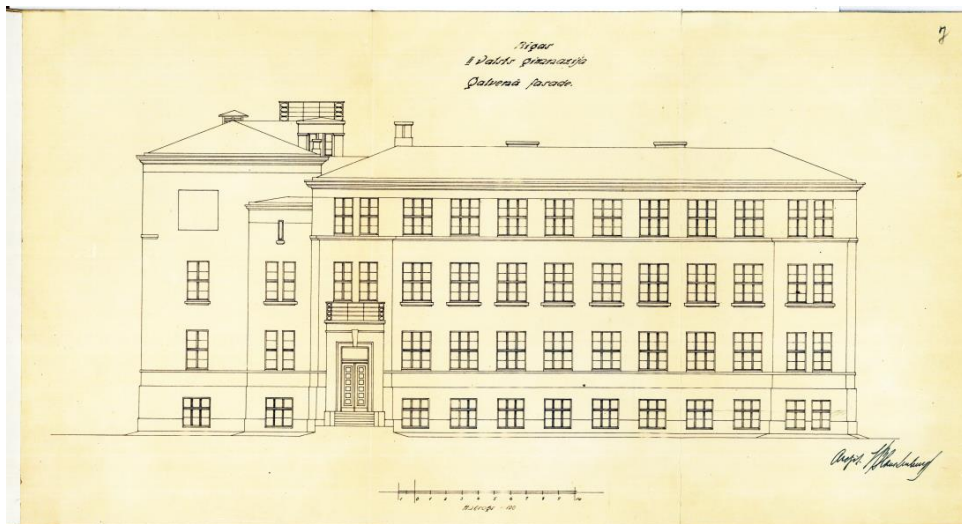
6.attēls. I.Blankenburga parakstītais Rīgas II Valsts ģimnāzijas, galvenās fasādes projekts [22].
